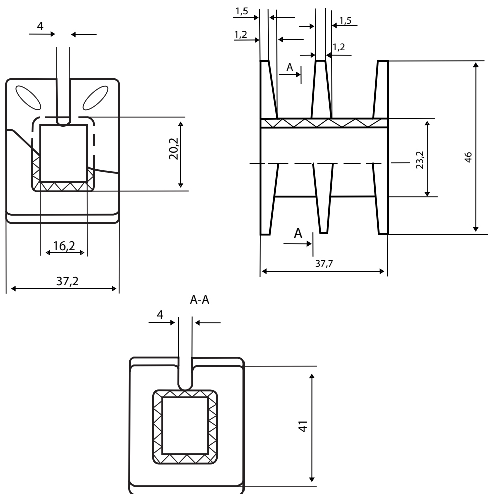
Габаритный чертеж
